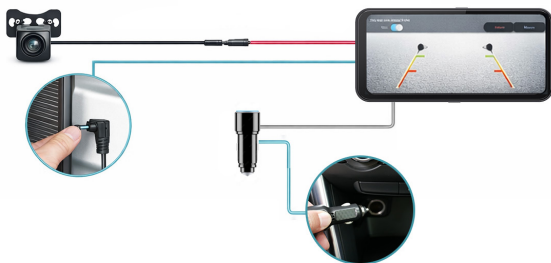
kamera cofania
