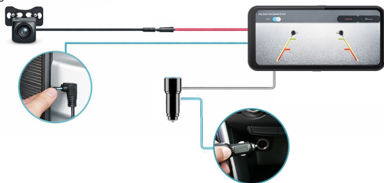
tagurduskamera
